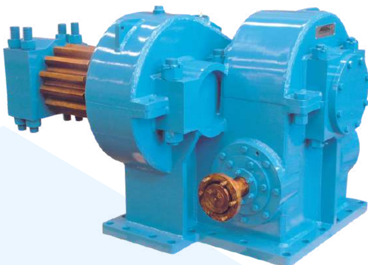
Acionamento carro torpeda (Siderurgia)
