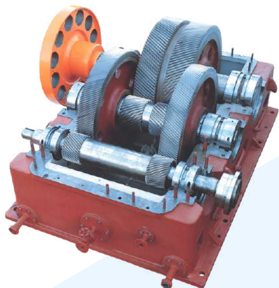
Redutor de alta para acionamento 2 ternos de moenda 34" x 66"
