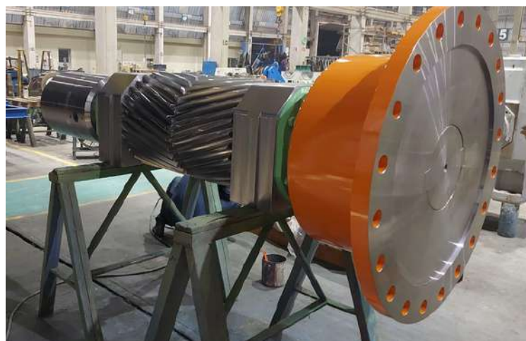
EIXO PINHÃO BI-HELICOIDAL PARA CAIXA DE TRANSMISSÃO DO LAMINADOR
