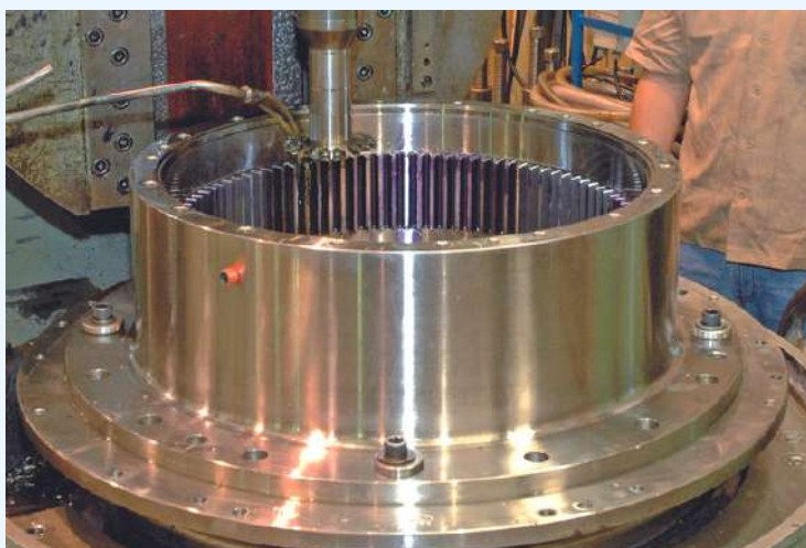
Anel dentado redutor planetário
